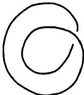
شکل ۱. نوار موبیوس ۱
