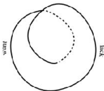
شکل ۳. میل/فقدان ۲
